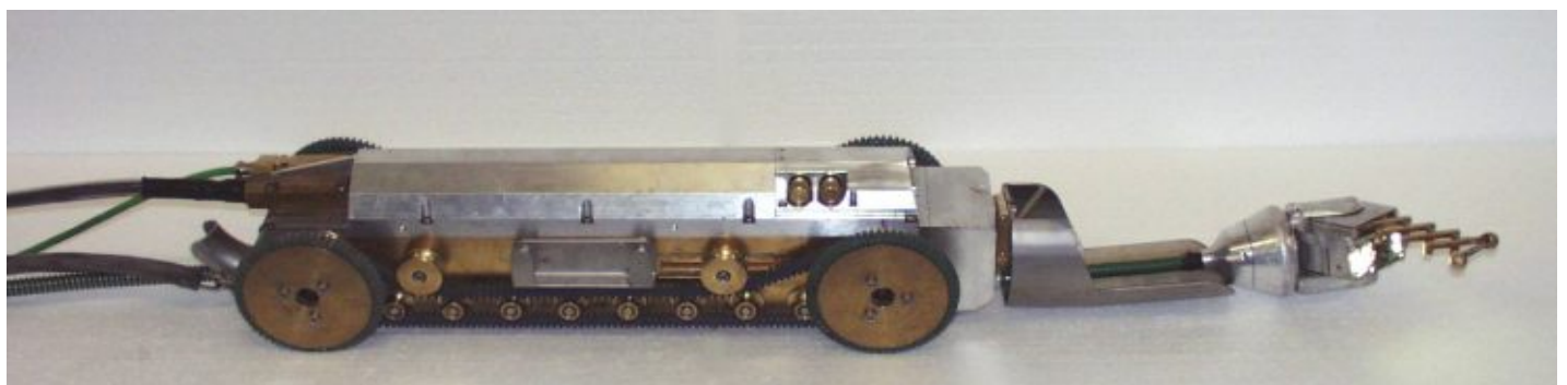
"Lindauer Schere" mit Fahrwagen
